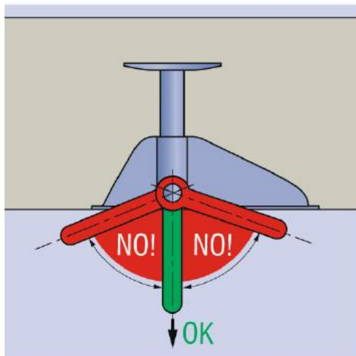
Abbildung 1 - Lastrichtung
