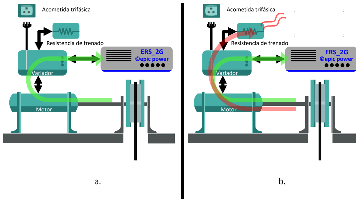
Fig. 4. Flujos de energía en regeneración
