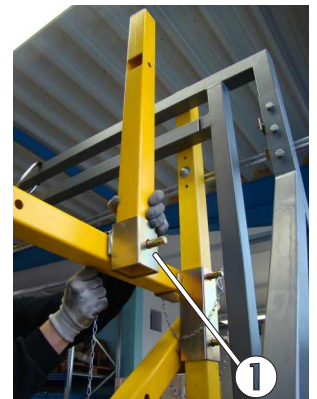
Bild 76: Positionierung des Aufnahmeteils inklusive oberer Geländerstütze
