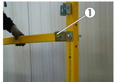
Bild 52: Steckbolzen zur Sicherung des Handlaufes
