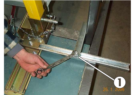
Bild 42: L-Profile zur Verankerung der Bühne zwischen der Türöffnung
