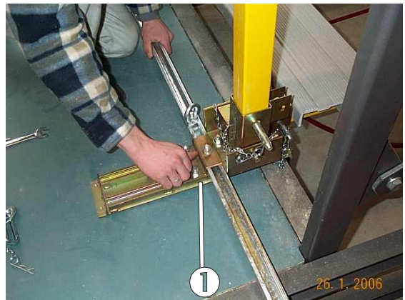
Bild 18: Fixierung der Quertraverse
