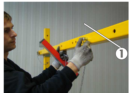
Bild 60: Fixierung von Innen- und Außenrohr mit einem kurzen Bolzen
