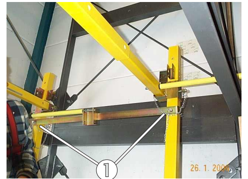
Bild 67: Befestigung des Adapters
