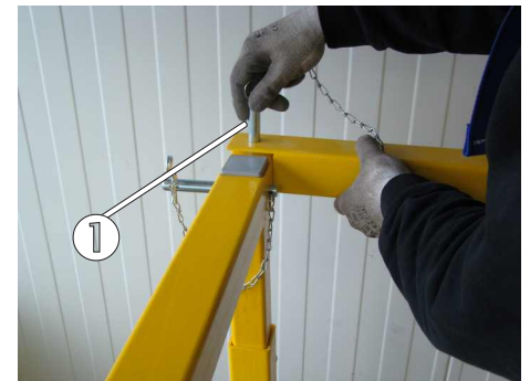
Bild 88: Der Steckbolzen wird zur Sicherung von oben eingeführt
