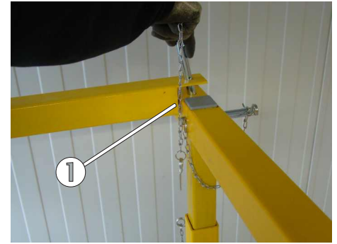
Bild 87: Auflegen und Sicherung des oberen stirnseitigen Handlaufes
