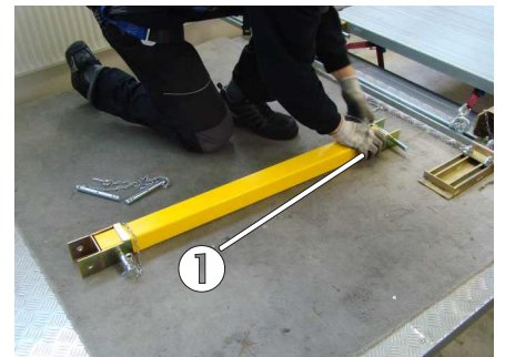
Bild 49: Vormontage des stirnseitigen Handlaufes
