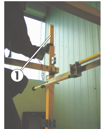
Bild 72: Hintere obere Geländerstütze
