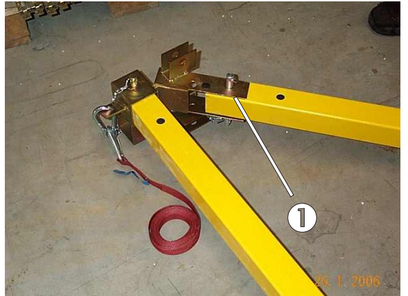
Bild 9: Fixierung des diagonalen Profils
