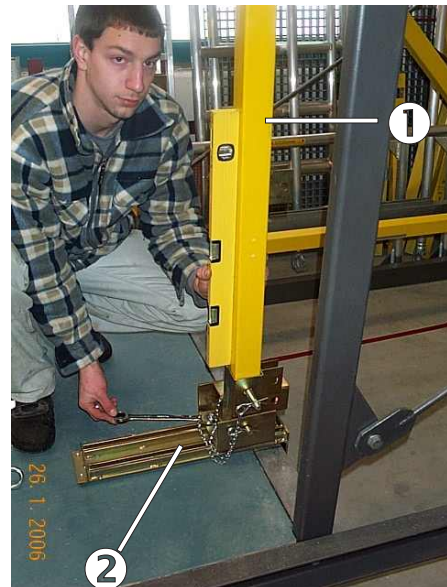
Bild 3: Vordere senkrechte Dreiecksseite In das montierte Schwellengelenk eingesteckt.
