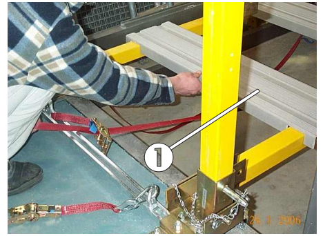
Bild 28: Ausrichten der vorderen Paneele
