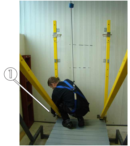
Bild 48: Sicherung mit kurzem Steckbolzen
