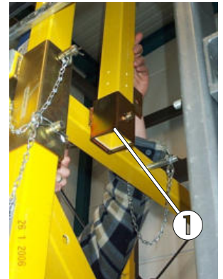
Bild 84: Positionierung des Aufnahmeteils inklusive oberer Geländerstütze
