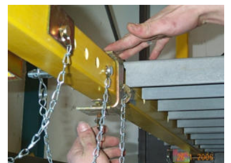
Bild 89: Rohrklemmen gegen das Verrutschen der Bodenpaneele
