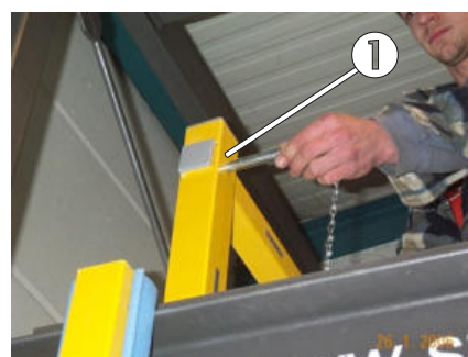
Bild 95: Das Innenrohr des Handlaufes wird in die vordere senkrechte Geländerstütze eingeführt und mit einem Bolzen gesichert
