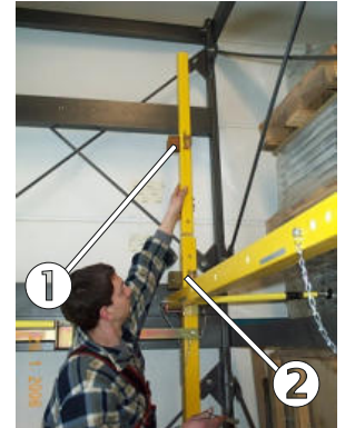
Bild 80: Hintere obere Geländerstütze
