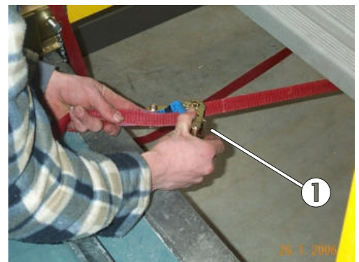
Bild 27: Mit Hilfe der Ratsche wird der Zurrurgurt auf geringe Vorspannung gebracht
