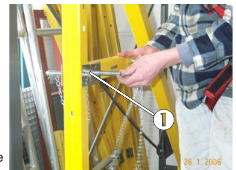
Bild 63: Auf das richtige Außenrohr muss geachtet werden
