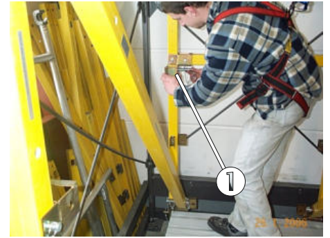
Bild 62: Montage der Kreuzhalter
