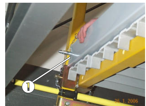
Bild 98: Sicherung der Fußleiste
