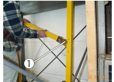
Bild 51: Montage des hinteren Handlaufes
