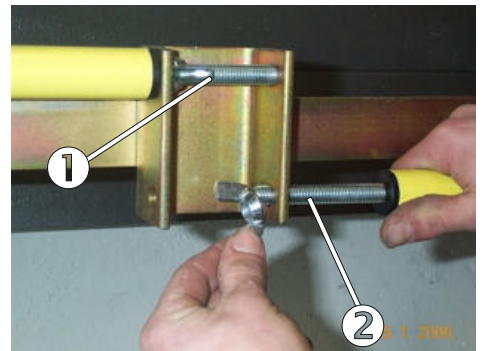
Bild 76: Befestigung der Teleskopstangen
