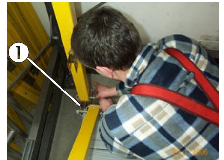
Bild 48: Sicherung mit kurzem Steckbolzen
