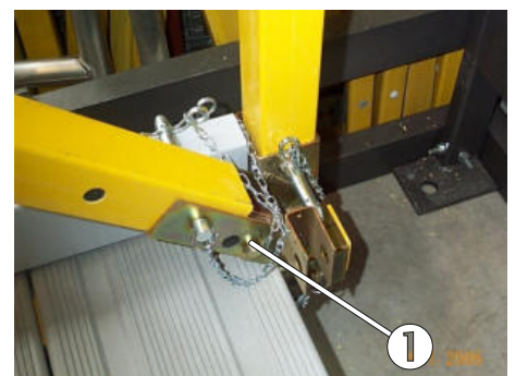
Bild 67: Fixierung der Fußleiste hinten mit einem langen Steckbolzen
