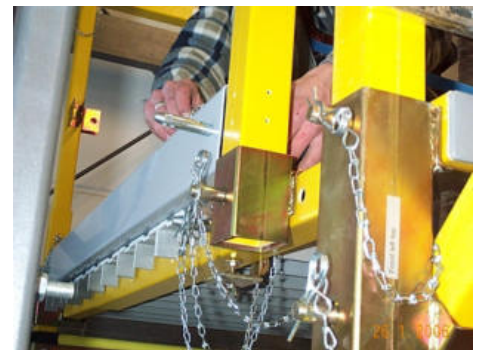
Bild 97: Der Steckbolzen wird zur Sicherung von oben eingeführt
