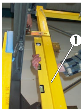
Bild 91: Ausrichten der Geländerstütze
