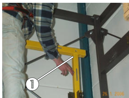
Bild 94: Das Außenrohr des Handlaufes wird über die hintere senkrechte Geländerstütze aufgesteckt
