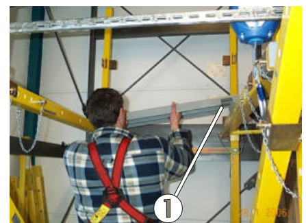
Bild 85: Auflegen der oberen Bodenpaneele
