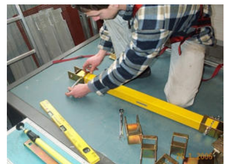
Bild 49: Vormontage des stirnseitigen Handlaufes
