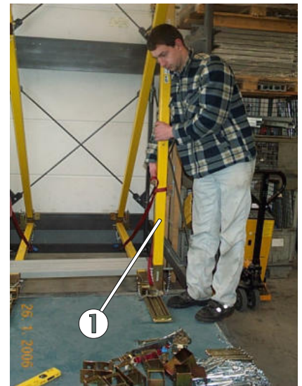
Bild 15: Anheben des Dreieckselementes
