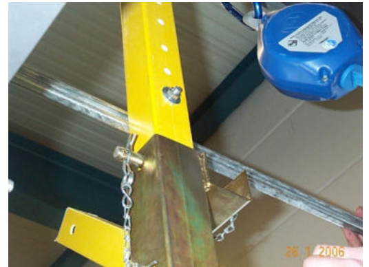
Bild 40: Fixierung der oberen Quertraverse
