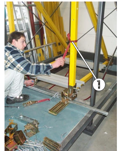
Bild 25: Lösen der zweiten Spanngurthälfte
