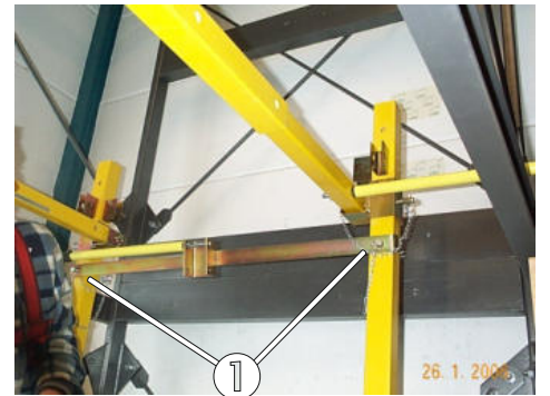
Bild 75: Befestigung des Adapters
