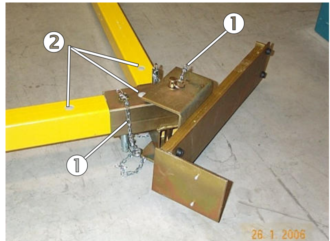
Bild 7: Kettenführung beachten.
