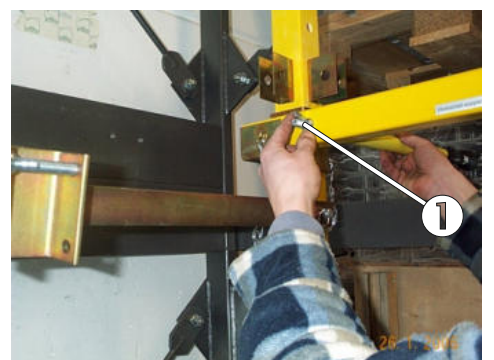
Bild 77: Alternative Befestigung der Teleskopstangen
