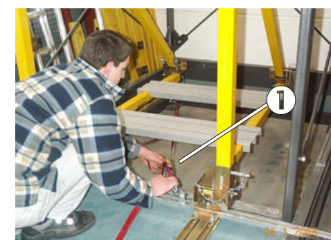
Bild 30: Gurte unter Vorspannung bringen
