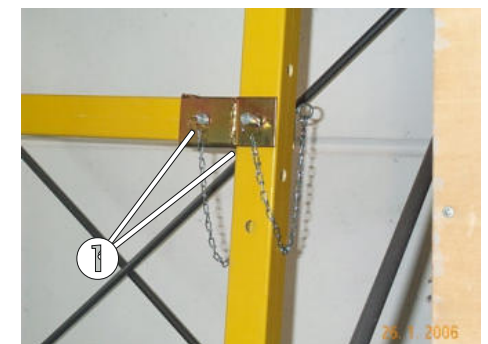
Bild 53: Gleichgerichtetes Stecken der Bolzen
