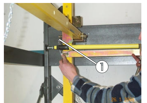
Bild 77: Alternative Befestigung der Teleskopstangen
