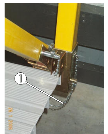
Bild 46: Bolzensicherung für die hintere senkrechte Geländerstütze
