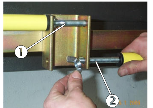
Bild 76: Befestigung der Teleskopstangen
