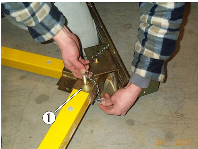
Bild 6: Senkrechte und waagrechte Dreiecksseite mit dem linken Schwellenwinkel verbunden
