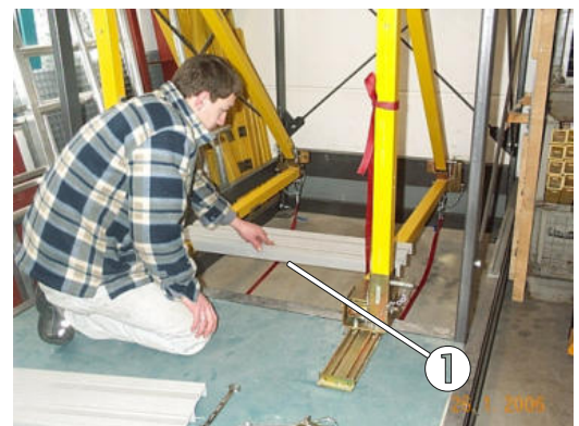
Bild 16: Erste Standardpaneel auflegen
