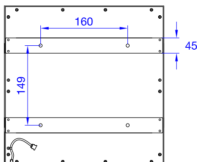
Rückansicht
